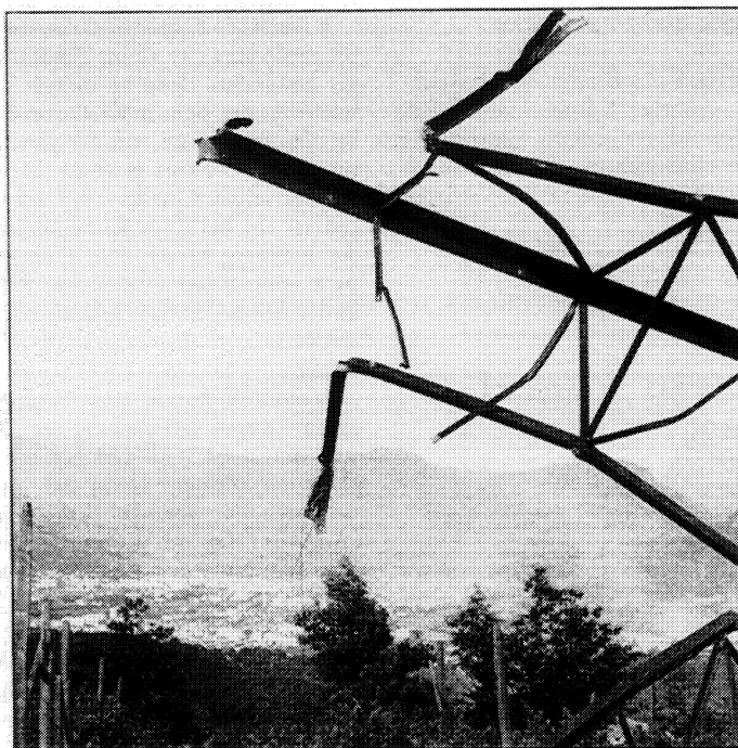
Elektromast bei Girlan 12.6.1961
